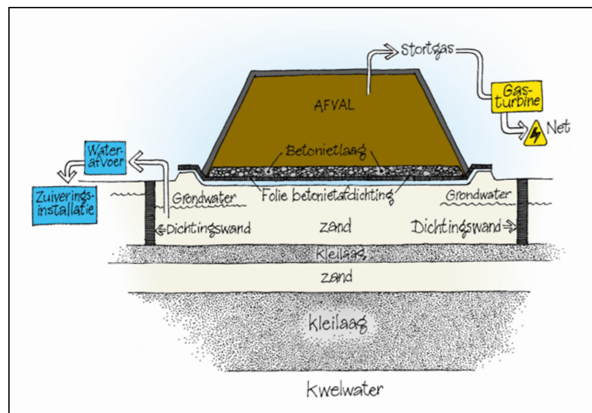
Dwarsdoorsnede stortlocatie
